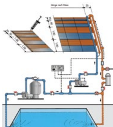
Solarpumpe
